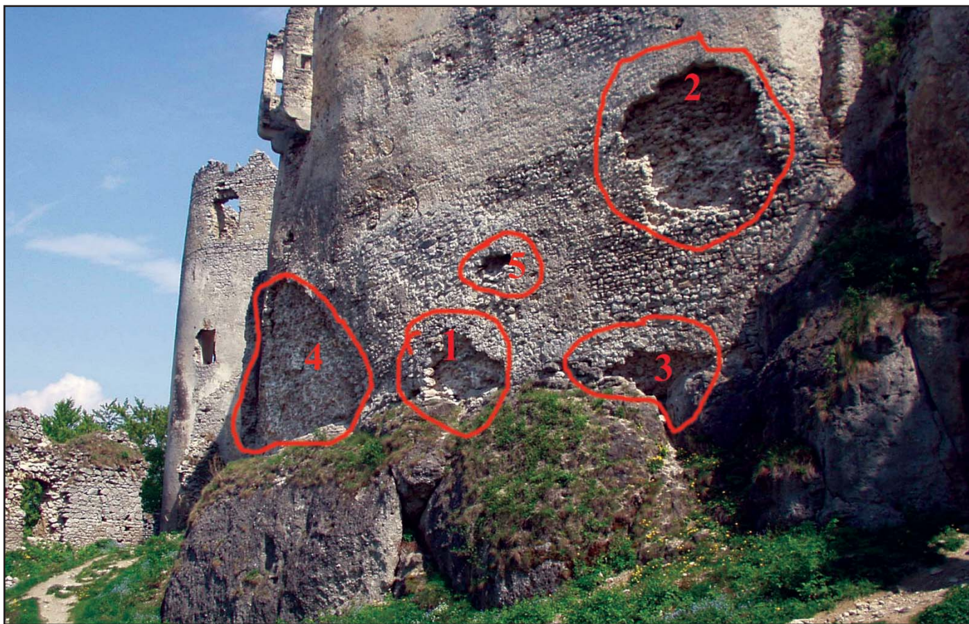
Porovnávací snímok plášťa SZ steny paláca. Hore: pred zásahom Dole: po vymurovaní kavern a doplnení malty v líci muriva
