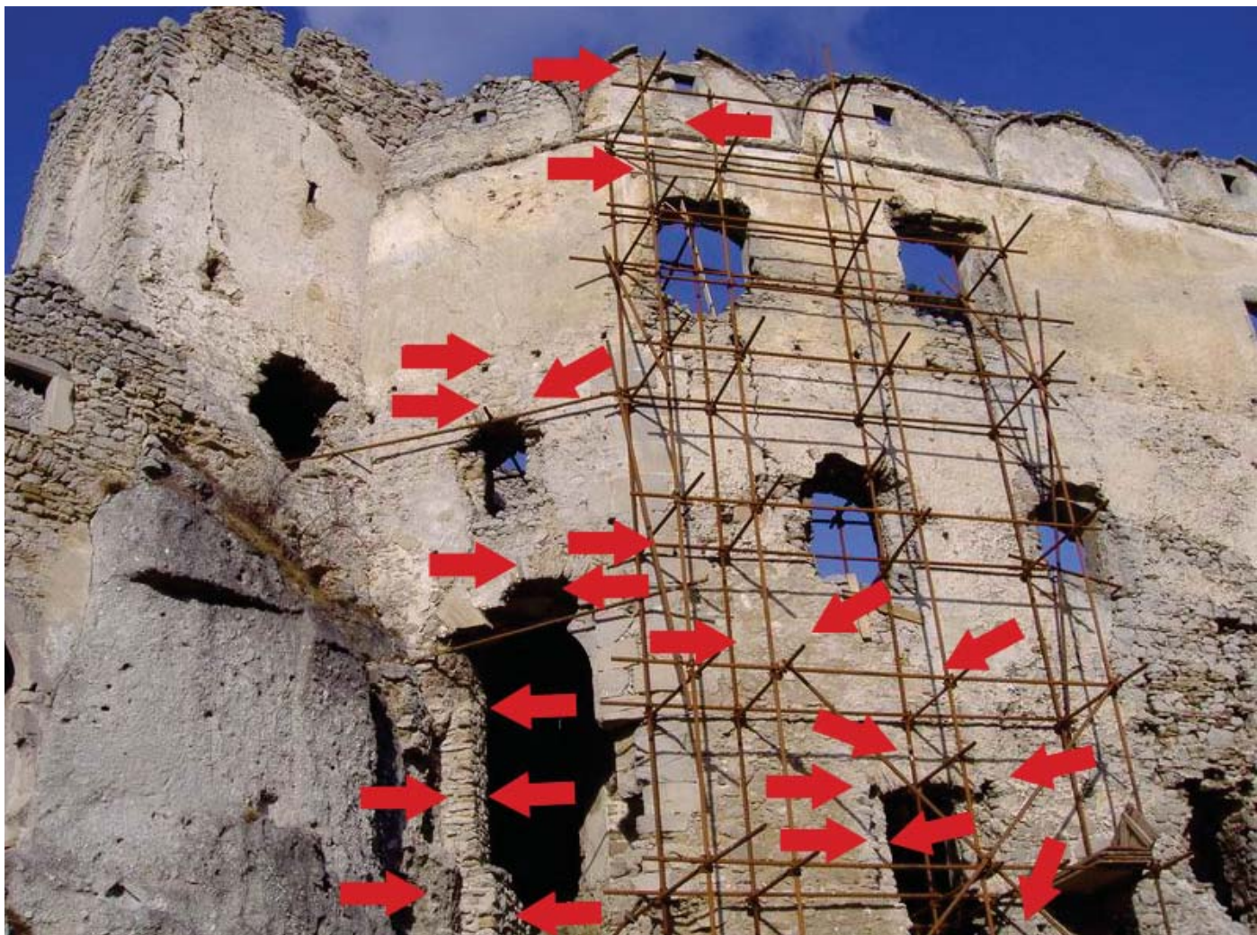
Snímok , ktorý vyznačenými šípkami znázorňuje miesta zásahov na juhovýchodnej stene paláca a taktiež ukazuje zásahy v priestore pôvodnej gotickej brány
